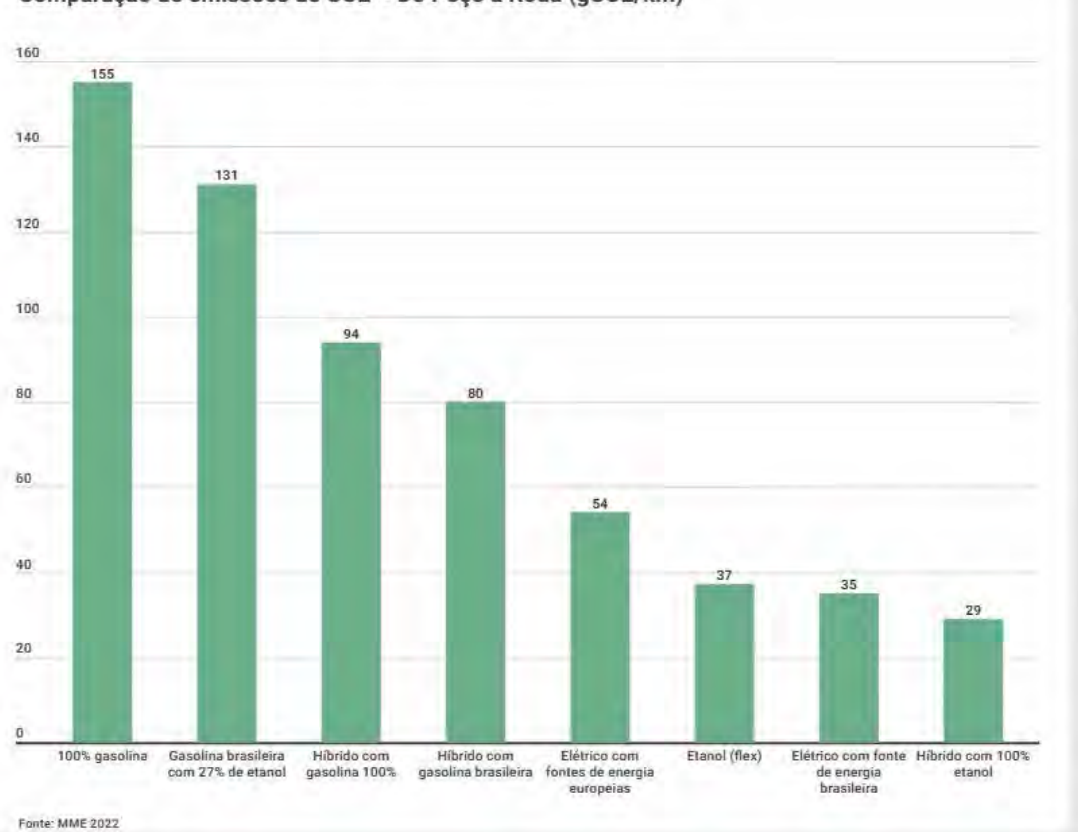
Comparação de emissões de CO 2 - Do Poço à Roda (gCO 2 /km)
