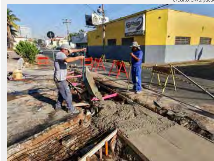
Construção de uma valeta de escoamento de água na Rua 8 com a Avenida 4
